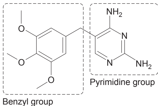
Trimethoprim
